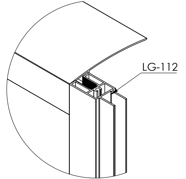
DETAY D ÖLÇEK 1 : 2
