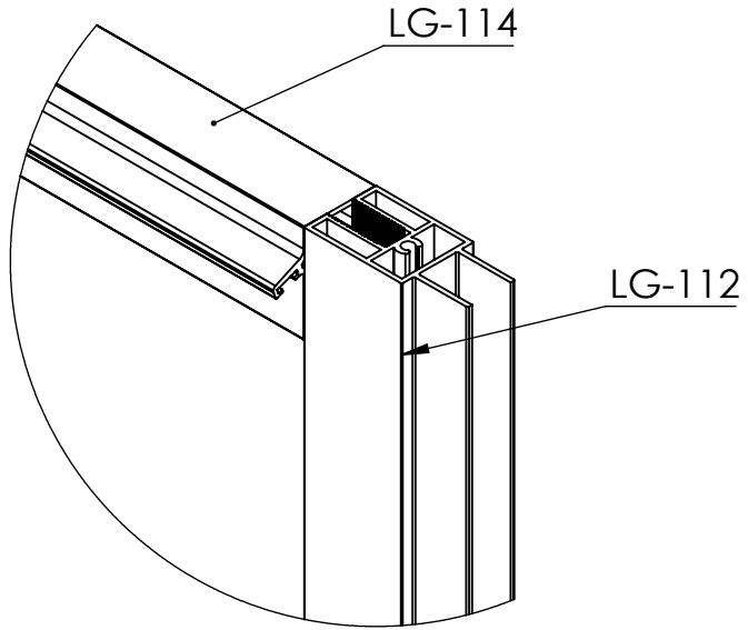
DETAY A ÖLÇEK 1 : 2
