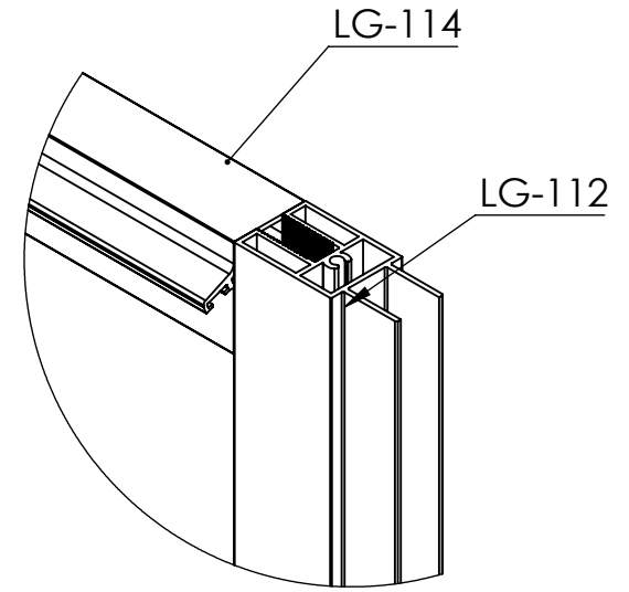
DETAY A ÖLÇEK 1 : 2
